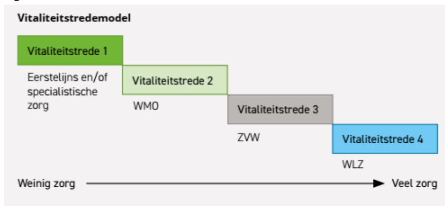
Figuur 0.1: Vitaliteitstredenmodel
