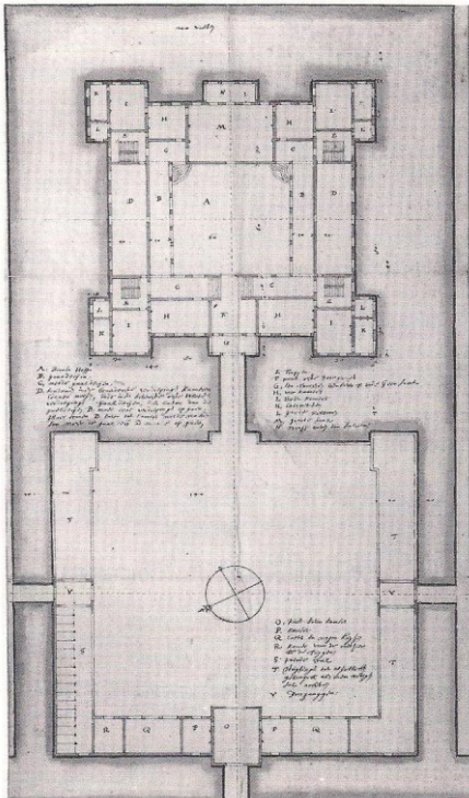
Ontwerptekening van kasteel Heeze door Pieter Post van 27 februari 1663.
