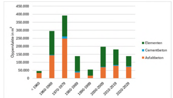
Afbeelding 7: verdeling areaal naar leeftijd, per type verharding
